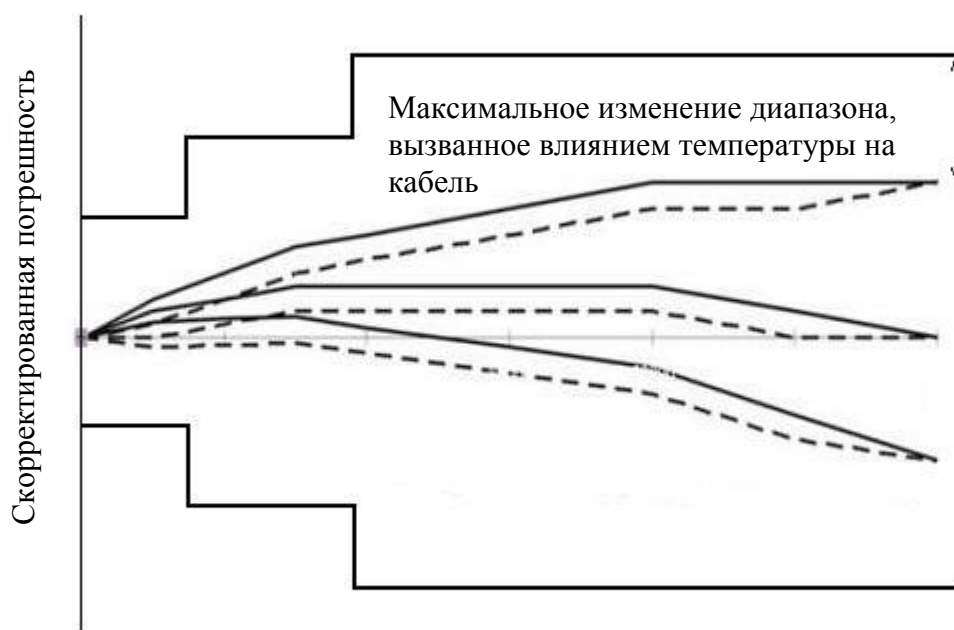
Рисунок 12 – Изменение диапазона из-за влияния температуры на кабель
